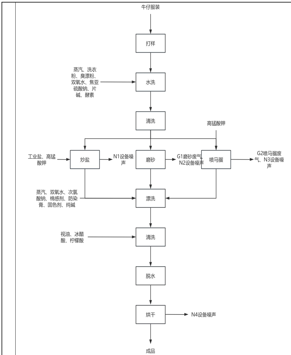
图 2-2 总工艺流程图
