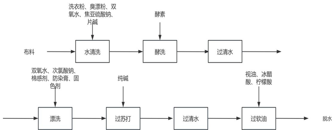
图 2-3 水洗工艺流程图
