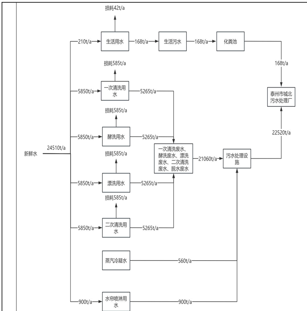
图 2-1 本项目水平衡图 (t/a)
