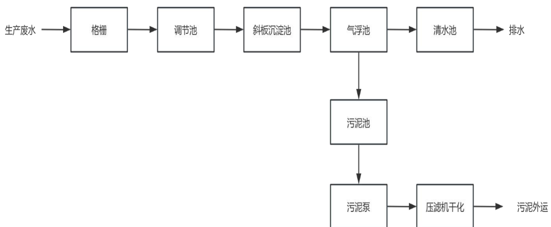
图 4-1 污水处理设施工艺流程
