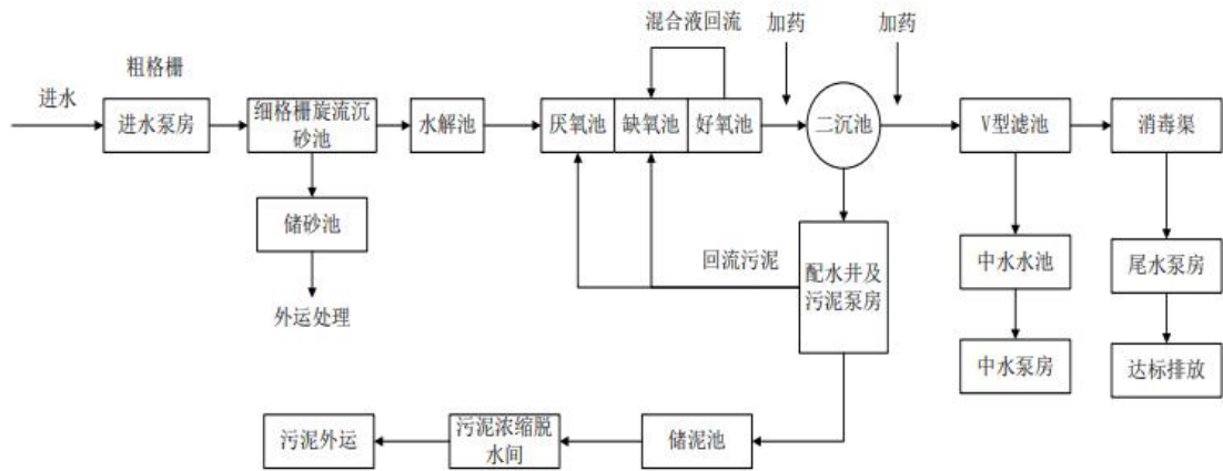
图 4-2 泰州市城北污水处理厂污水处理工艺流程
